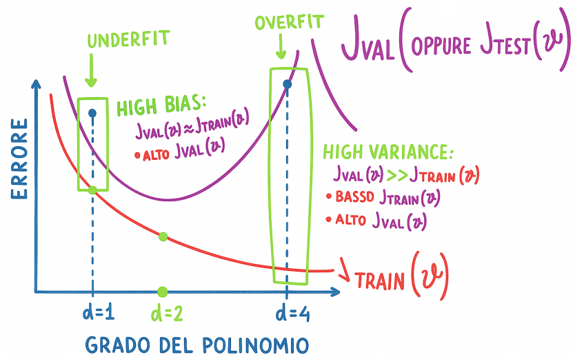
Figura 5.3: Trade-off tra bias e varianza in funzione della complessità del modello.
